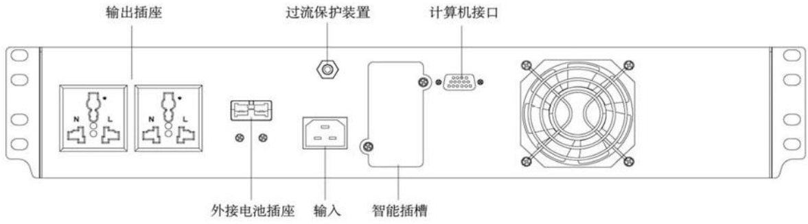
1KSR 机架式 UPS 后盖板示意图
