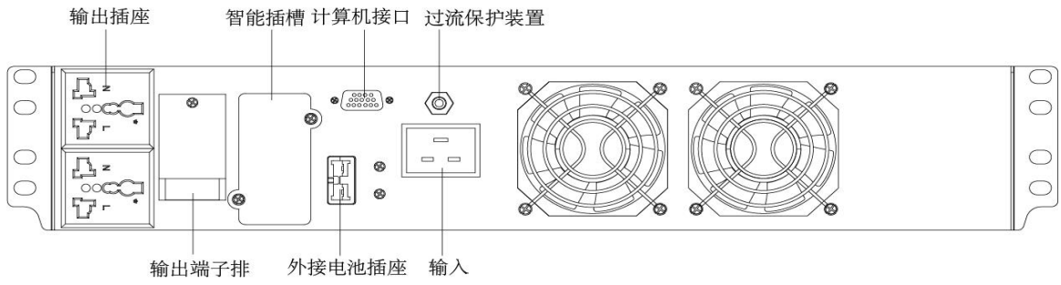
3KSR 机架式 UPS 后盖板示意图
