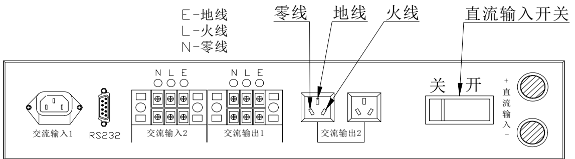
3, 4, 5, 6KVA 逆变电源后面板
