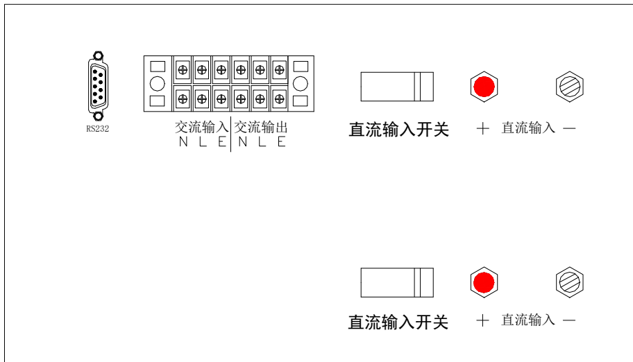
G 型机箱机械尺寸 单位: mm 误差: ±0.5
