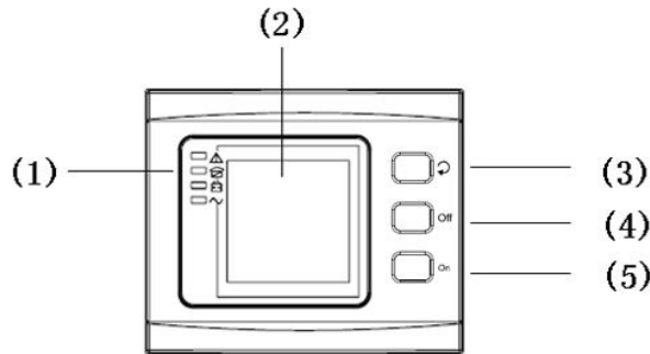
模块LCD面板部件说明图
