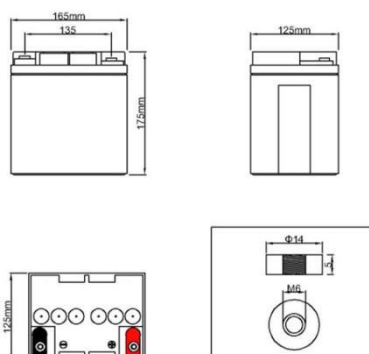
12V24Ah
