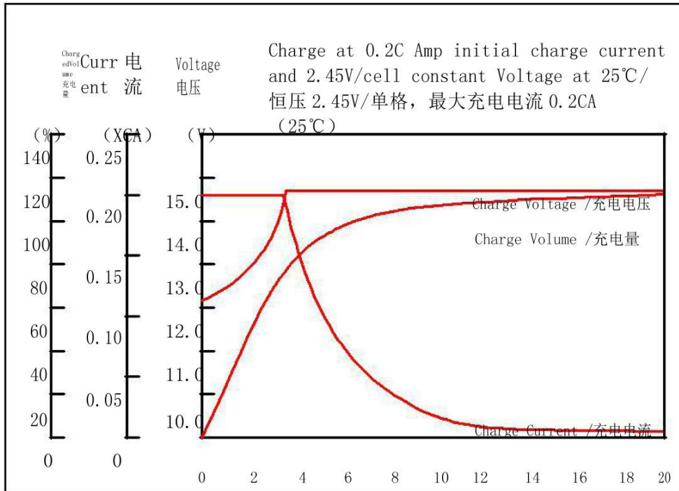
充电特性
