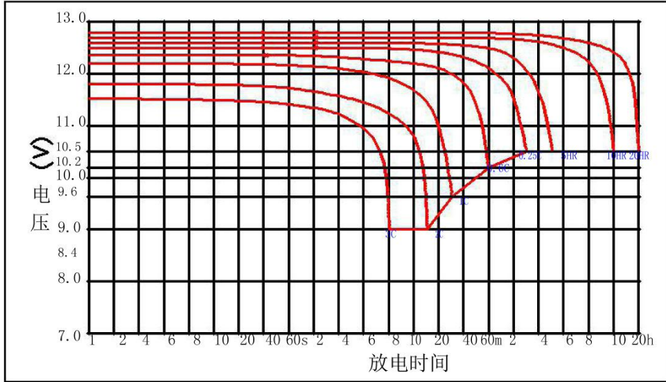
放电特性
