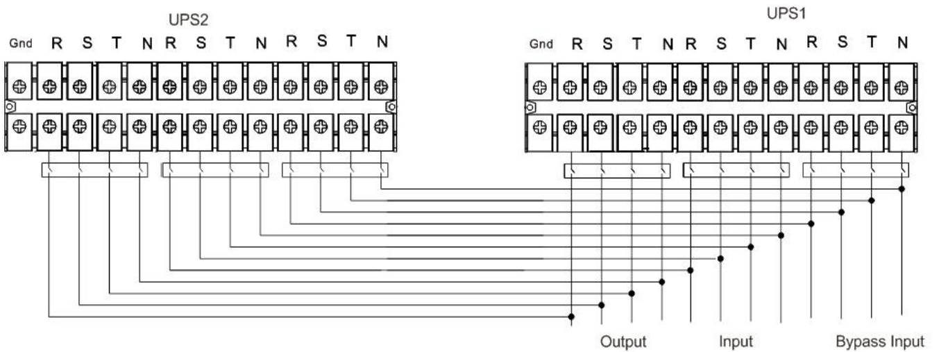
30K(S)/40K(S) 双输入并机系统接线图
