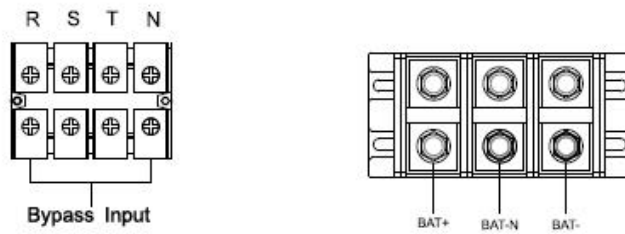
60KS/80KS 双输入端子排示意图
