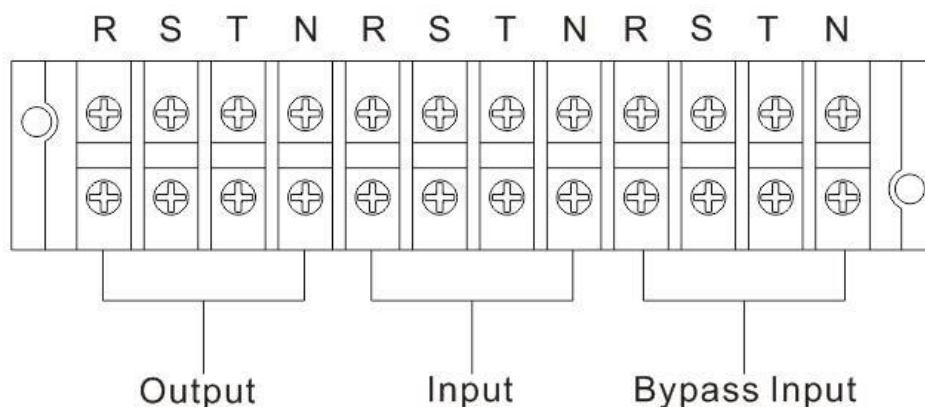
10K(S)/15K(S)/20K(S) 端子台示意图
