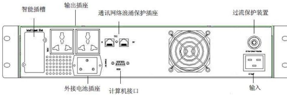
DT1K(S) RACK UPS 后盖板示意图
