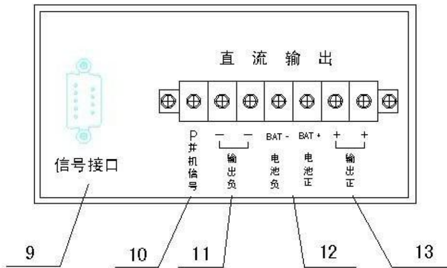
电源输出端局部放大图
