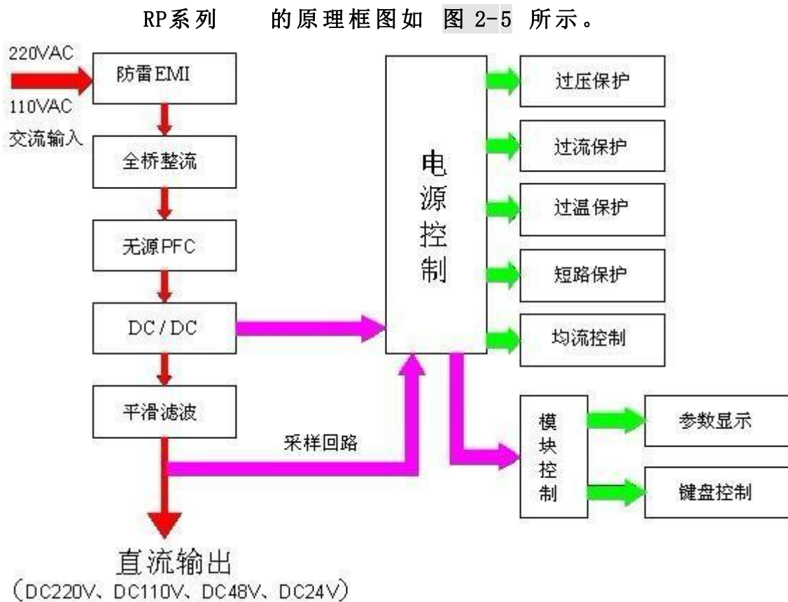
图 2-5 RP系列原理框图
