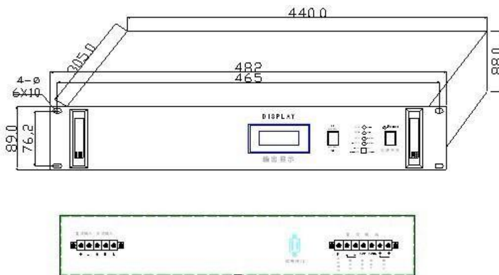
图 1-1 RP 系列 外形示意图
