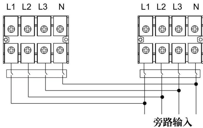
60K 并机接线图
