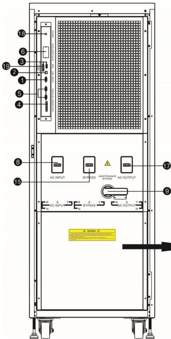
图 8: 180K /200K 前 面板
