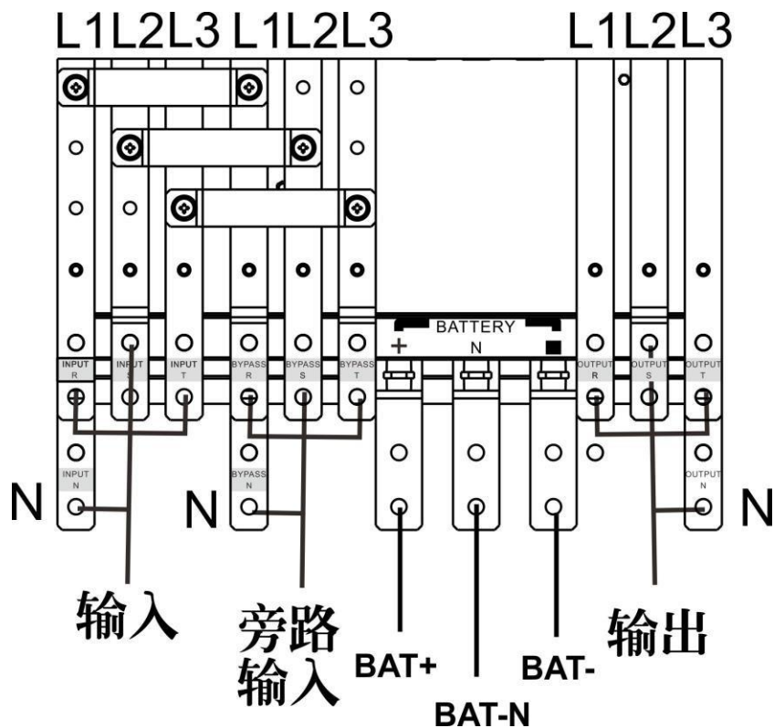
100K / 120K / 180K / 200K 接线端子示意图
