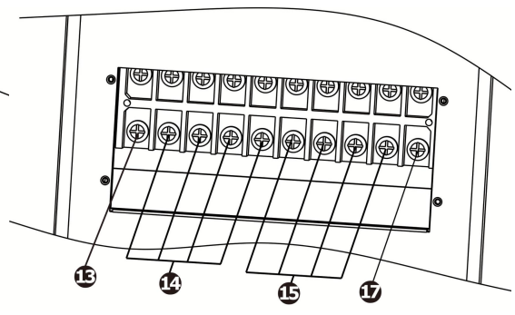
图 5: 30K(S) 输入/输出端子台
