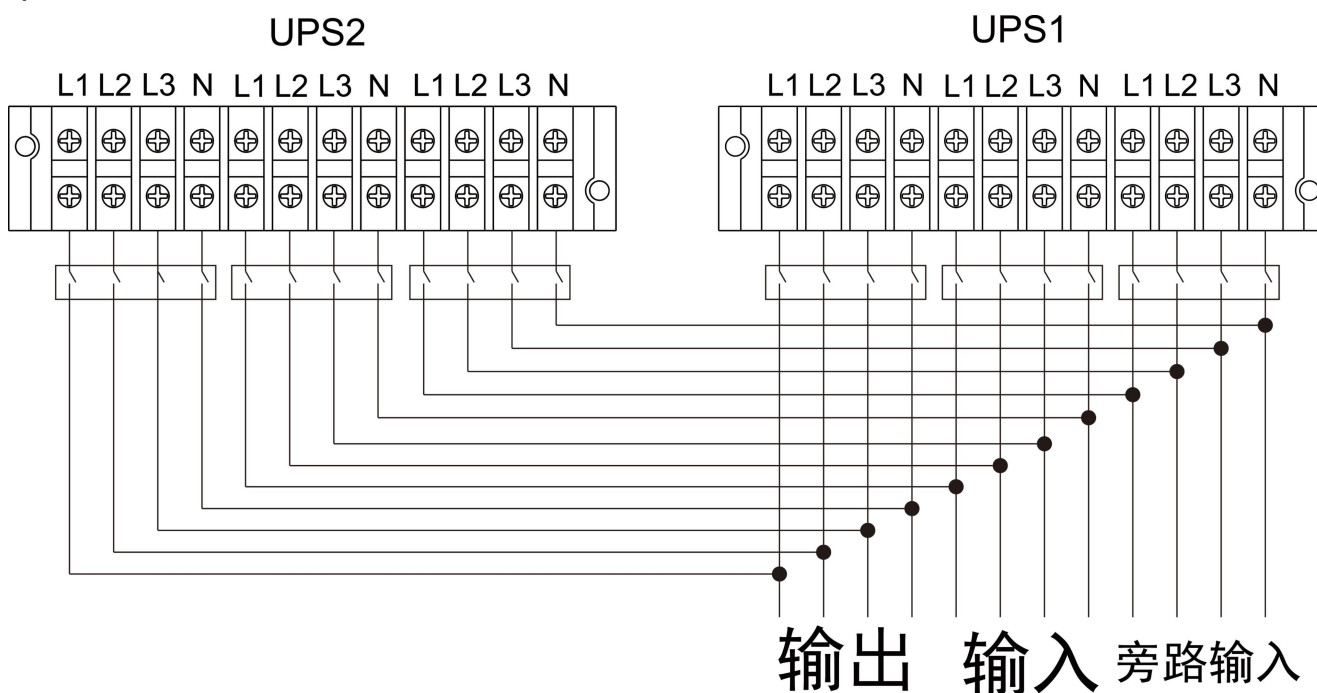
10K (L) ,20K(S)并联系统布线图
