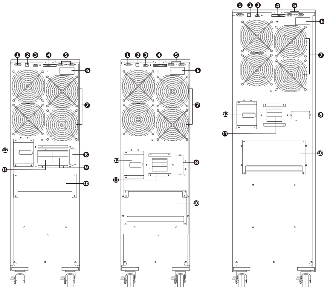
图 1: 10K(S)/15K(S)/20K(S)背板图 图 2: 30KL 背板图
