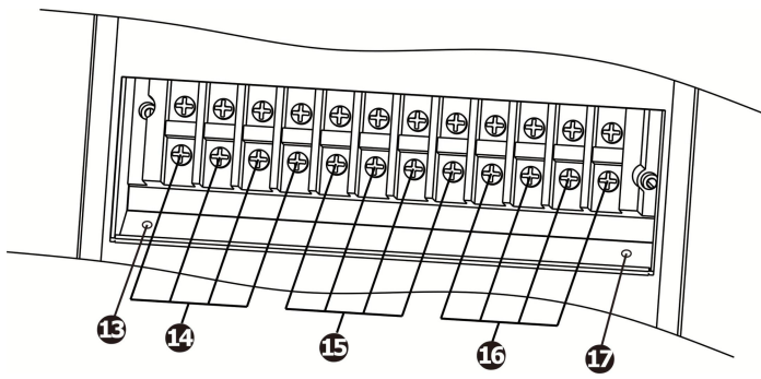
图 4: 10K(S)/15K(S)/20K(S) 输入/输出端子台
