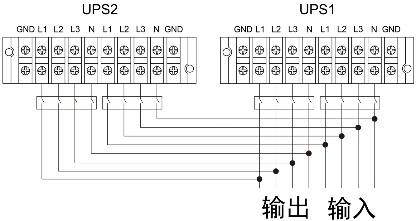
30K(S)并联系统布线图
