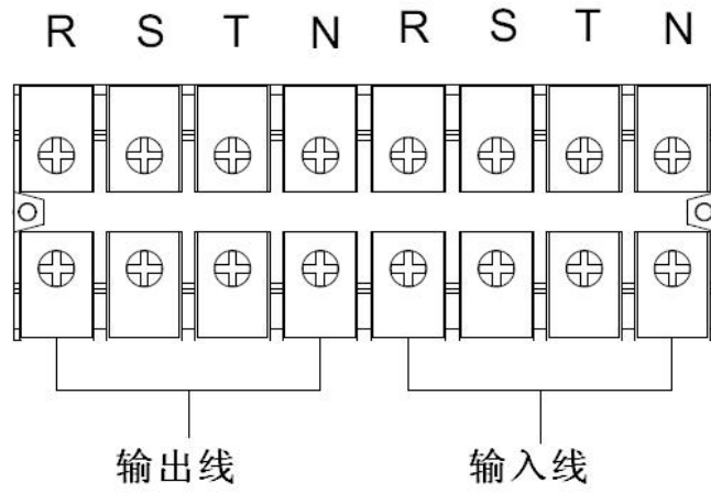
HV 30K(L)/40K(L)端子台示意图
