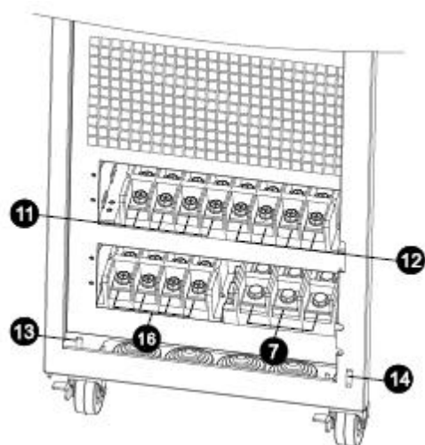
图 12: 60KL/80KL 双输入
