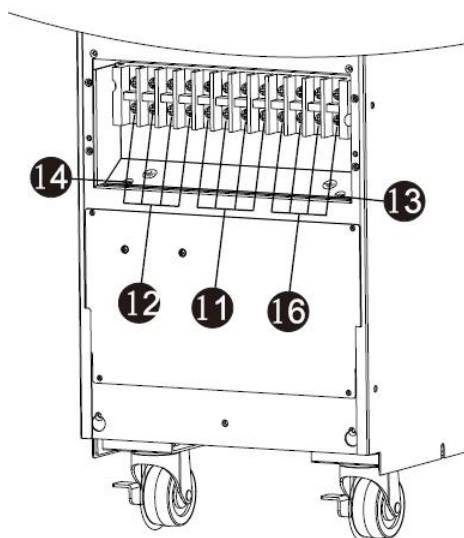
图 4: 10K(L)/15K(L)/20K(L) 双输入 输入/输出端子台
