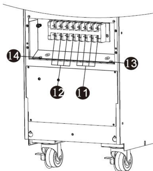
图 3: 10K(L)/15K(L)/20K(L) 输入/输出端子台
