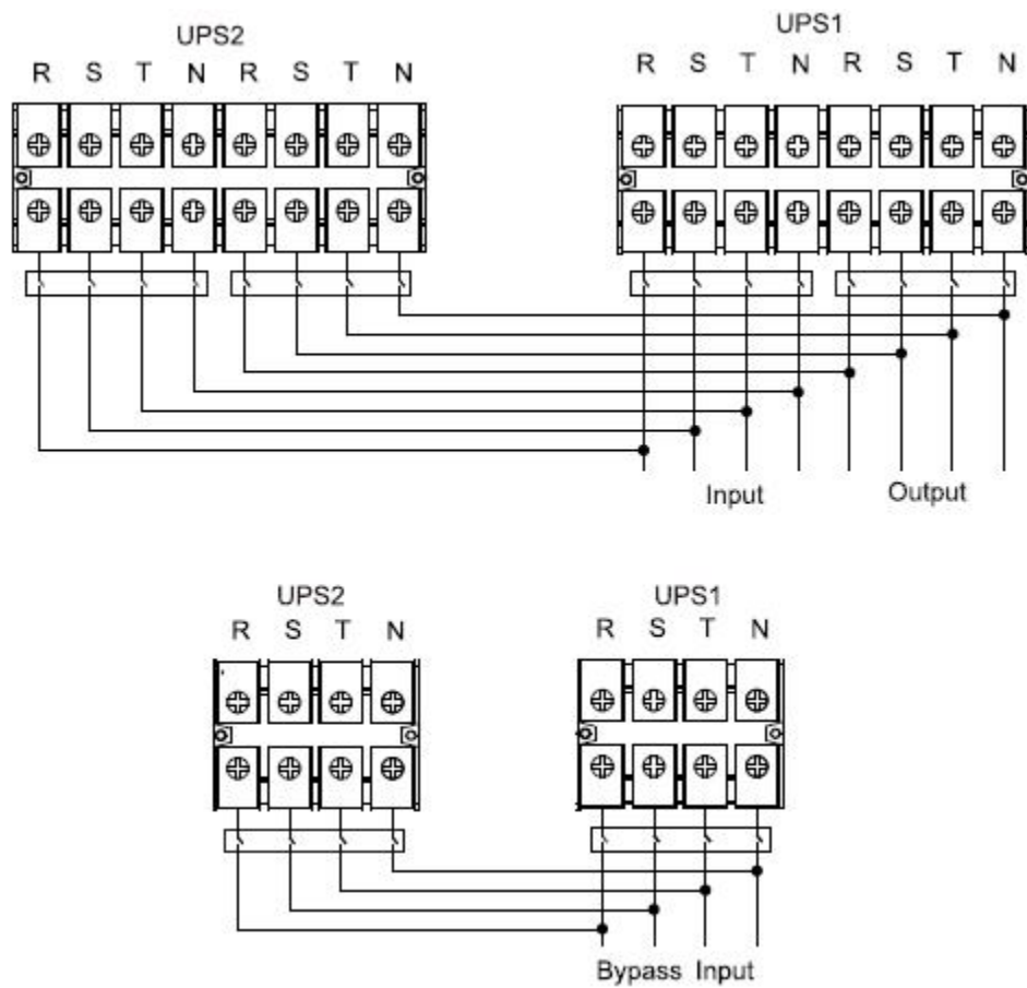
HV 60KL/80KL 双输入并机系统接线图
