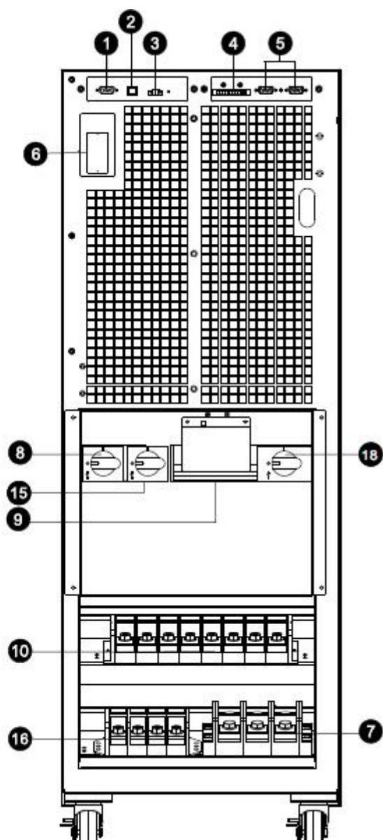
图 10: 80KL
