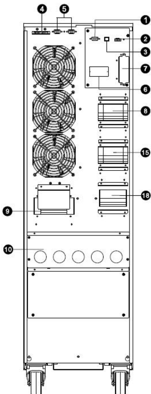
图 5: 30K(L)/40K(L) 后背板
