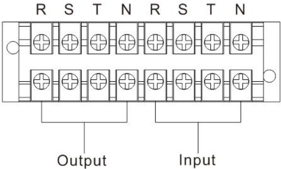
HV10K(L)/15K(L)/20K(L) 端子台示意图
