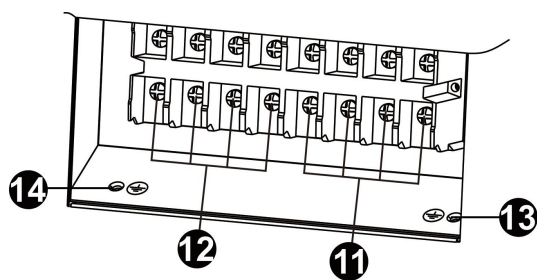
图 7: 30K(L)/40K(L) 输入/输出端子台
