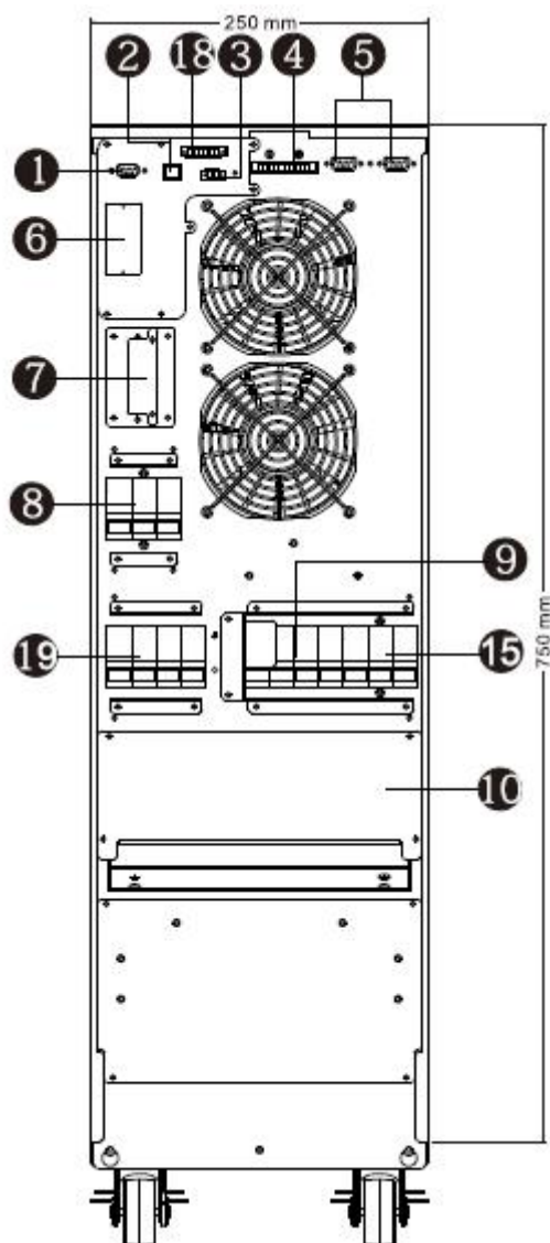
图 2: 10K(L)/15K(L)/20K(L) 双输入后背板
