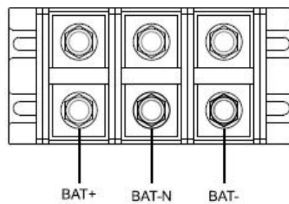
HV 60KL/80KL 端子排示意图
