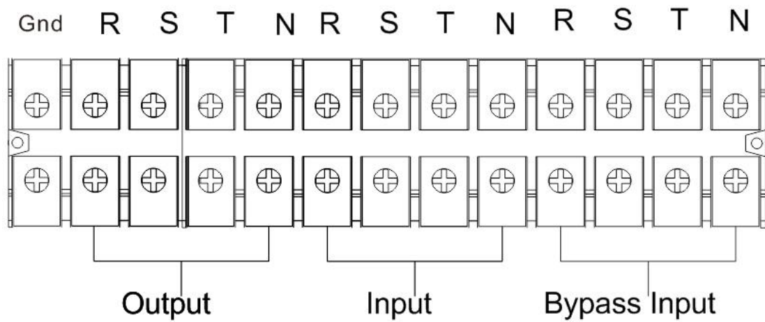
双输入 HV 30K(L)/40K(L)端子排示意图
