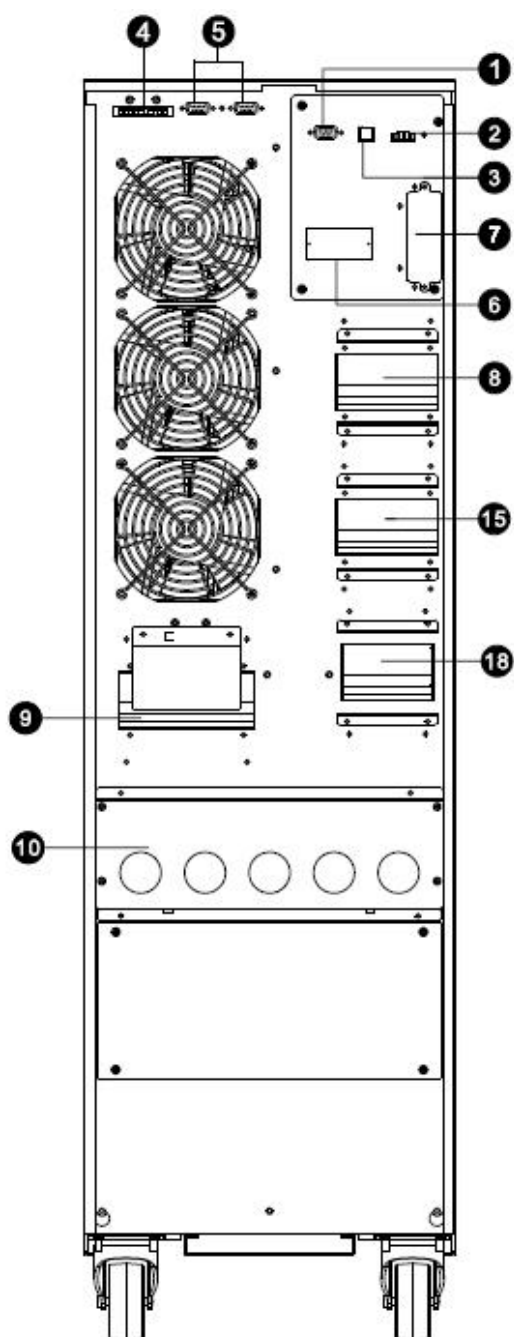
图 6: 30K(L)/40K(L) 后背板
