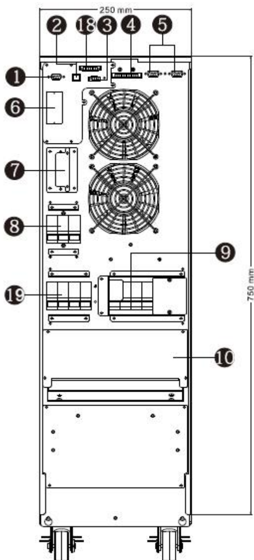
图 1: 10K(L)/15K(L)/20K(L) 后背板
