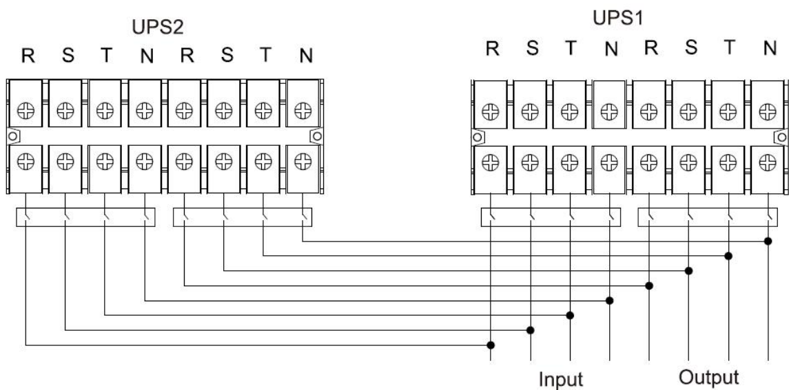
HV 60KL/80KL 并机系统接线图
