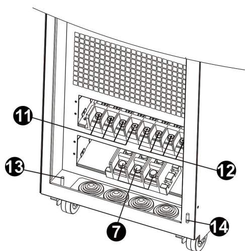
图 11: 60KL/80KL
