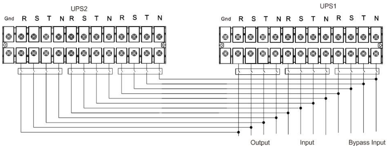
HV 30K(L)/40K(L) 双输入并机系统接线图
