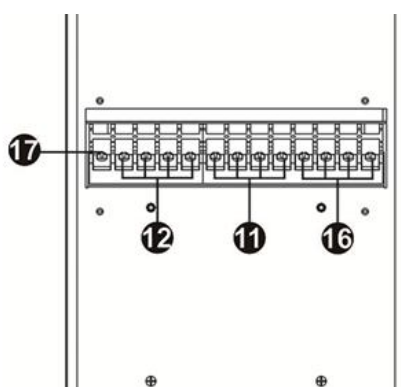
图 8: 30K(L)/40K(L) 双输入 输入/输出端子台
