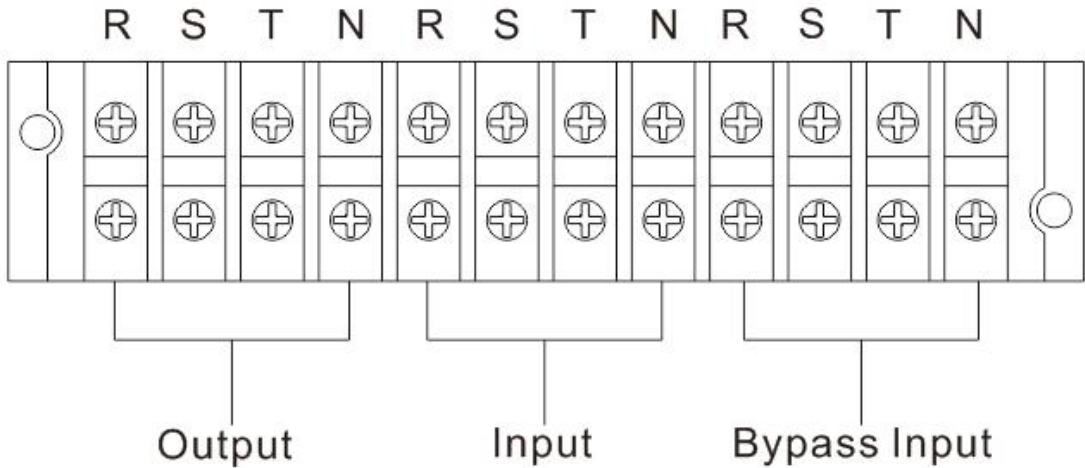
双输入 HV10K(L)/15K(L)/20K(L) 端子台示意图
