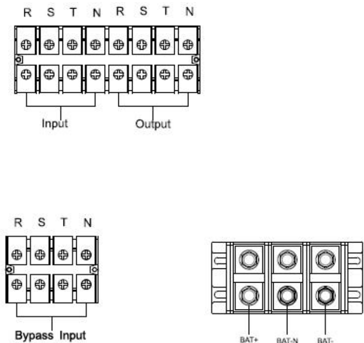
HV 60KL/80KL 双输入端子排示意图
