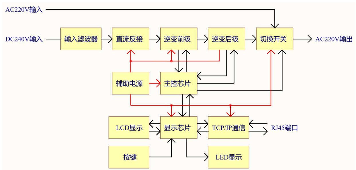
原理框图
