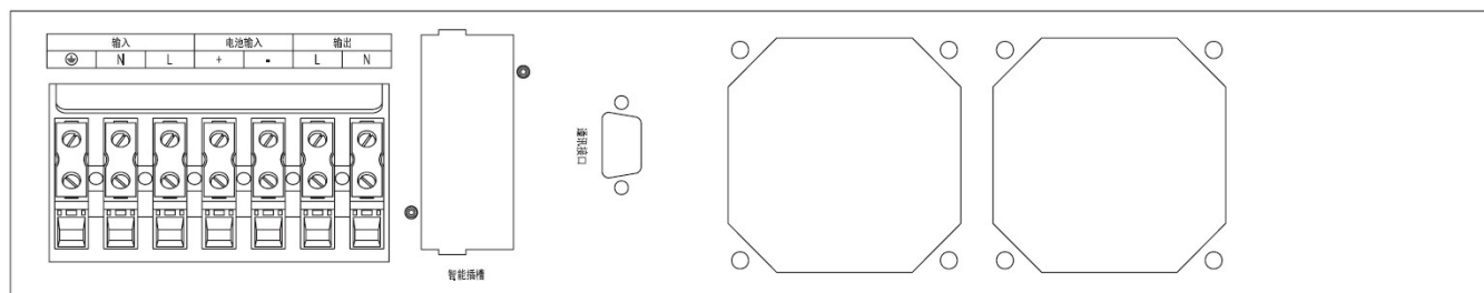
E3KS 机架式 UPS 后盖板示意图
