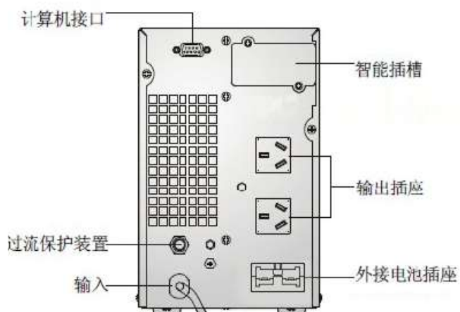
1K 后盖板
