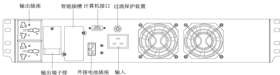
ET3KRS 机架式 UPS 后盖板示意图
