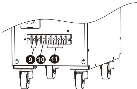
图 3: 10KXL 输入输出端子
