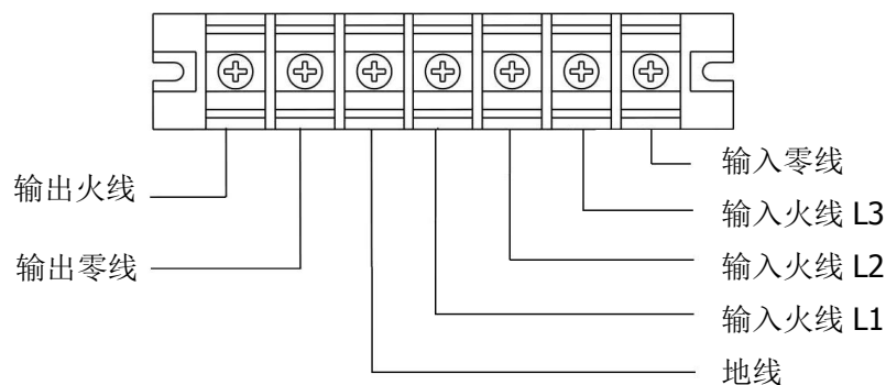
端子台示意图
