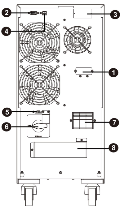
图 1:10KXL 背面面板
