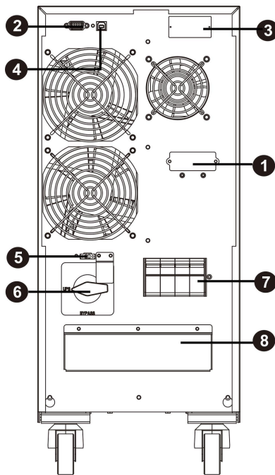
图 2:15KXL/20KXL 背面面板
