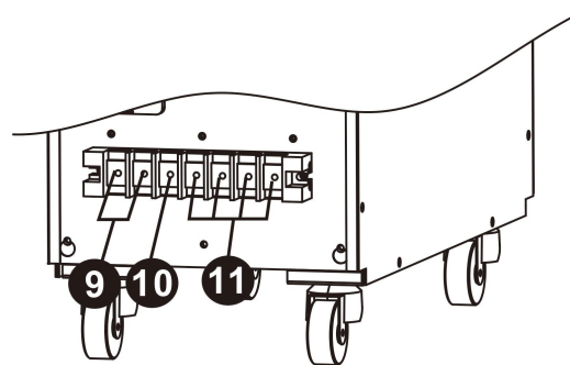
图 4: 15KXL/20KXL 输入输出端子
